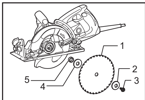
► 1. Lame 2. Bague externe 3. Boulon hexagonal 4. Bague interne 5. Bague 17
