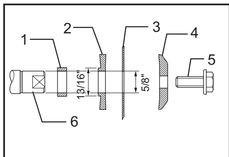
► 1. Bague 17 2. Bague interne 3. Fer 4. Bague externe 5. Boulon hexagonal 6. Axe de montage
